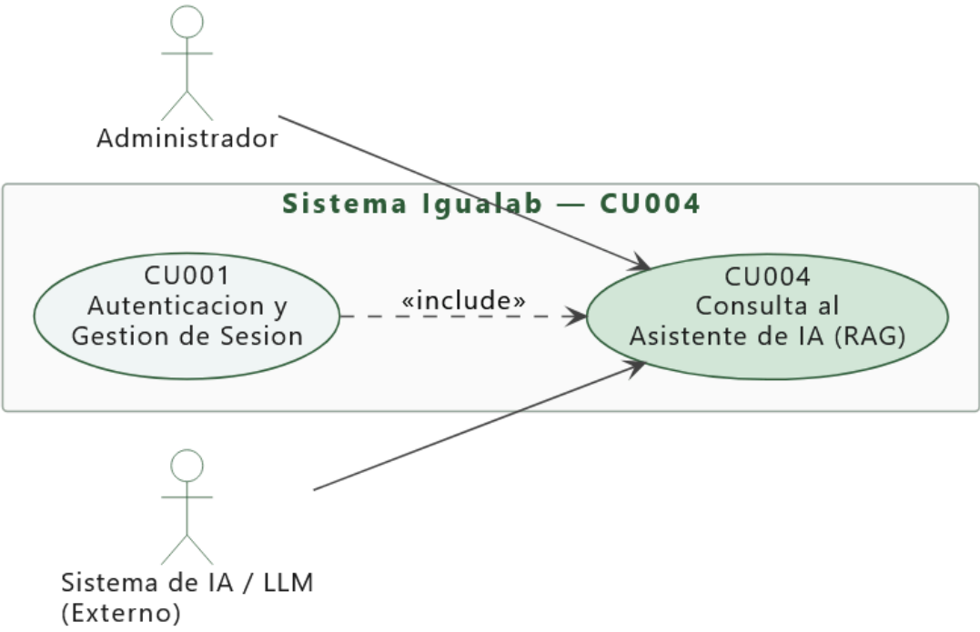
[ IMAGEN ] Diagrama de caso de uso — CU004
